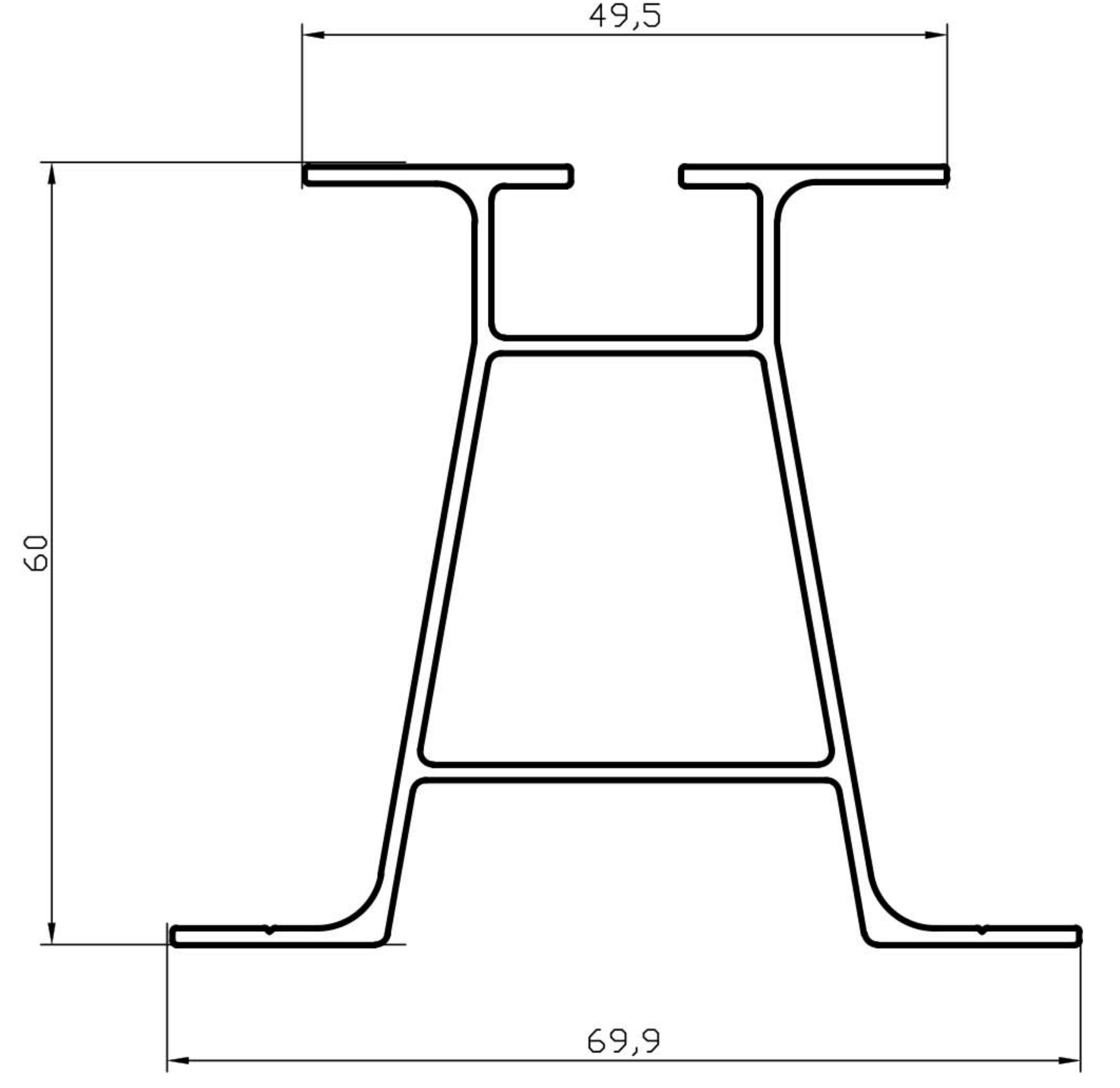
K-7615 879 gr/m
