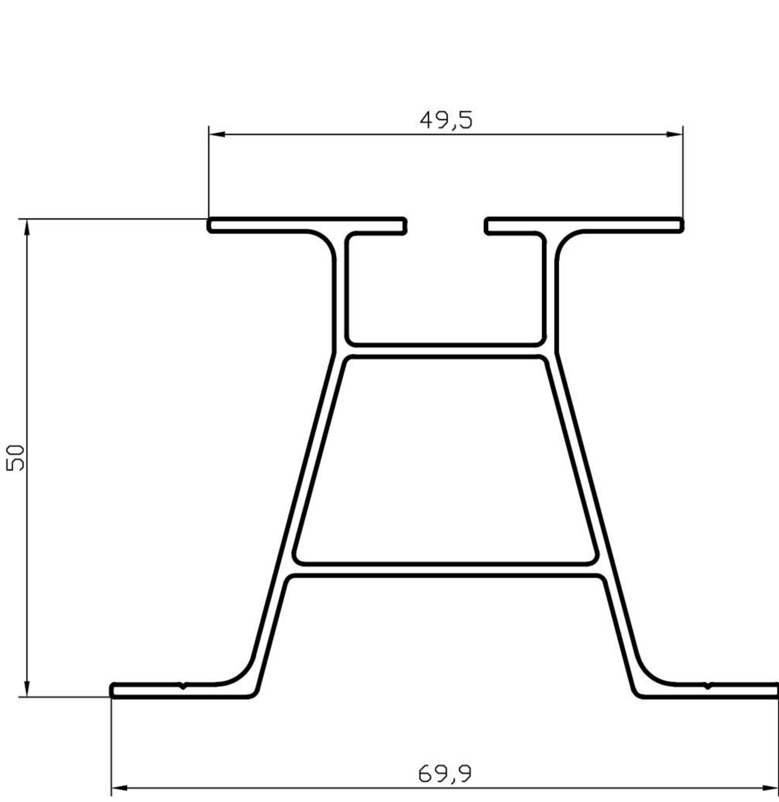
K-7610 799 gr/m
