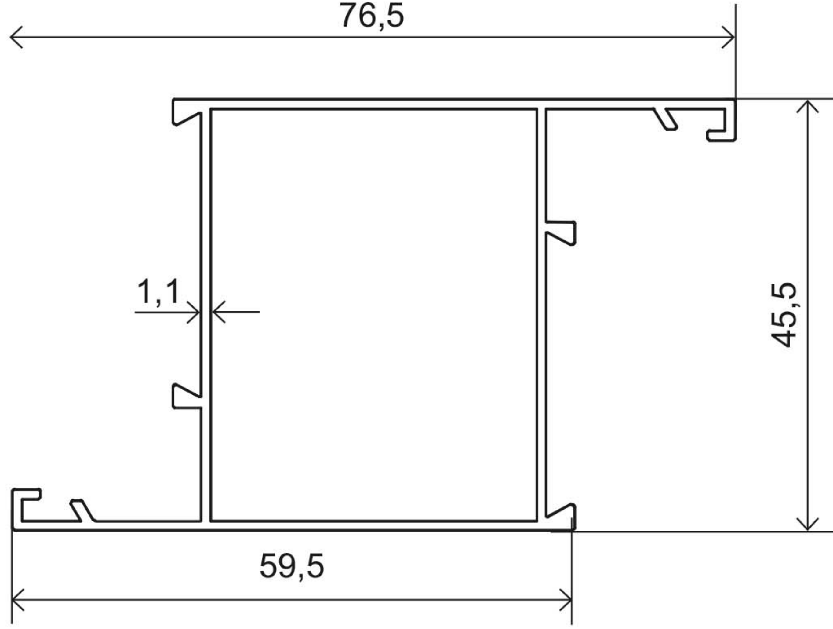
K-2060 650 gr/m
