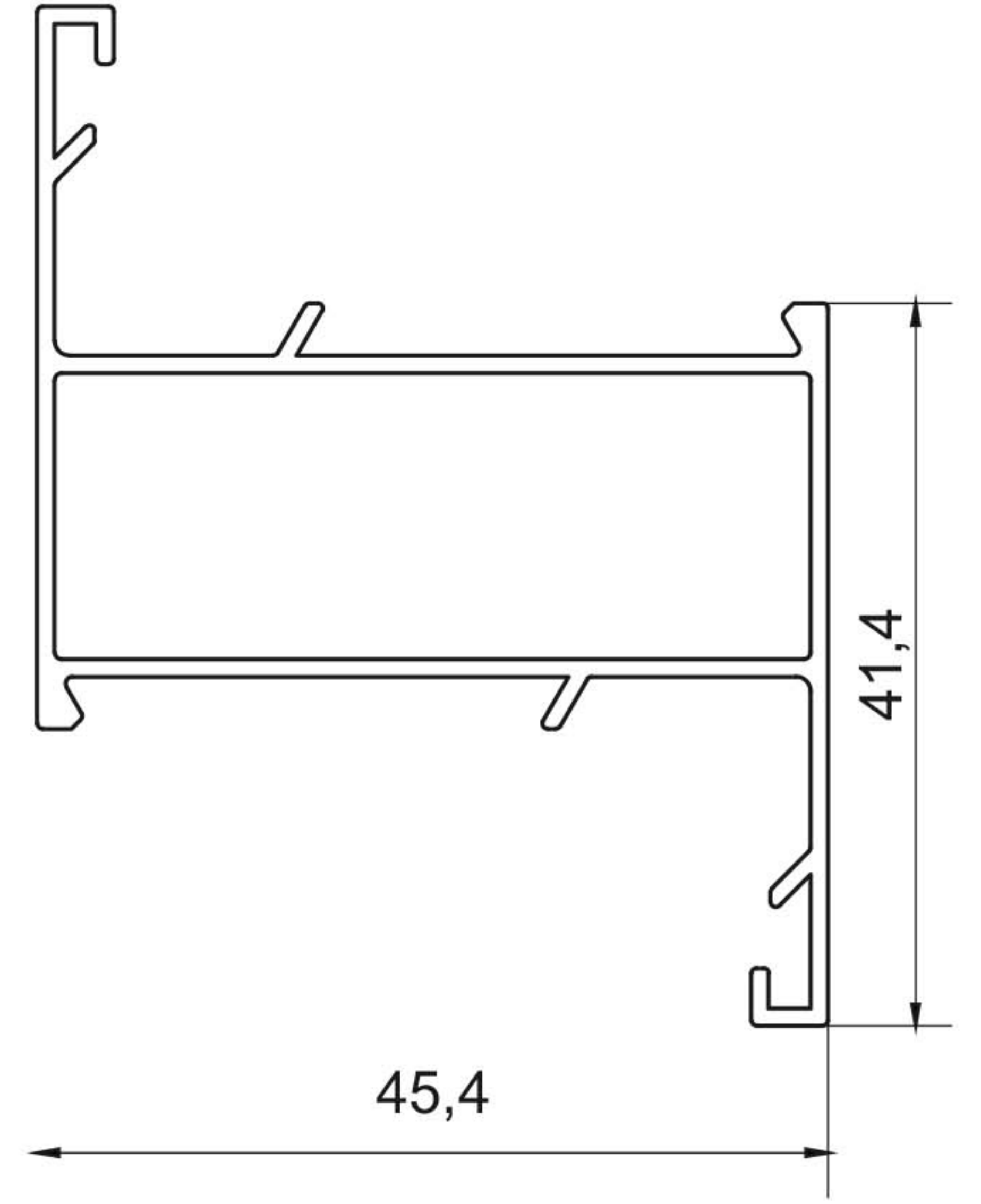
K-2045 545 gr/m
