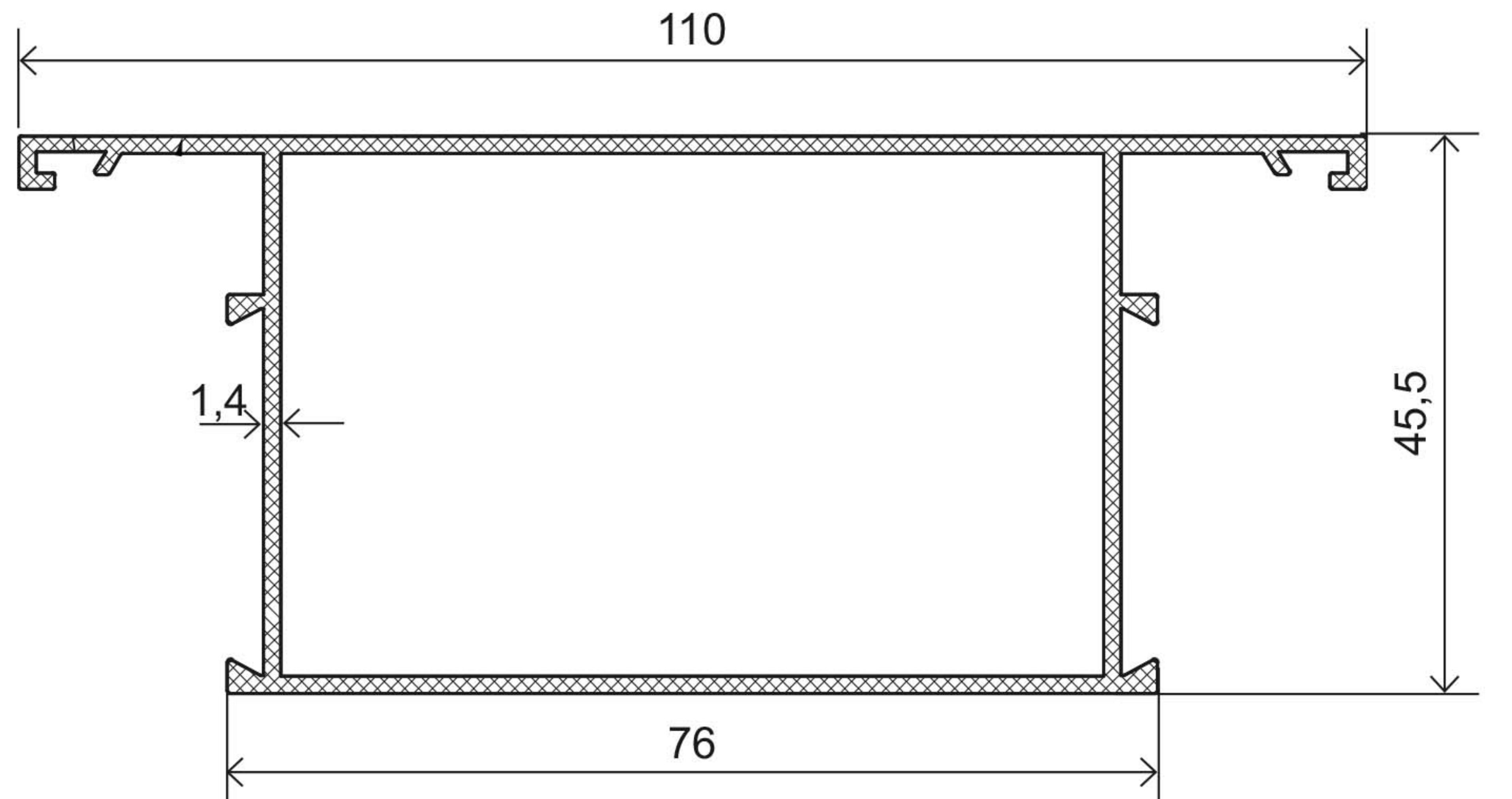
K-2050 1114 gr/m
