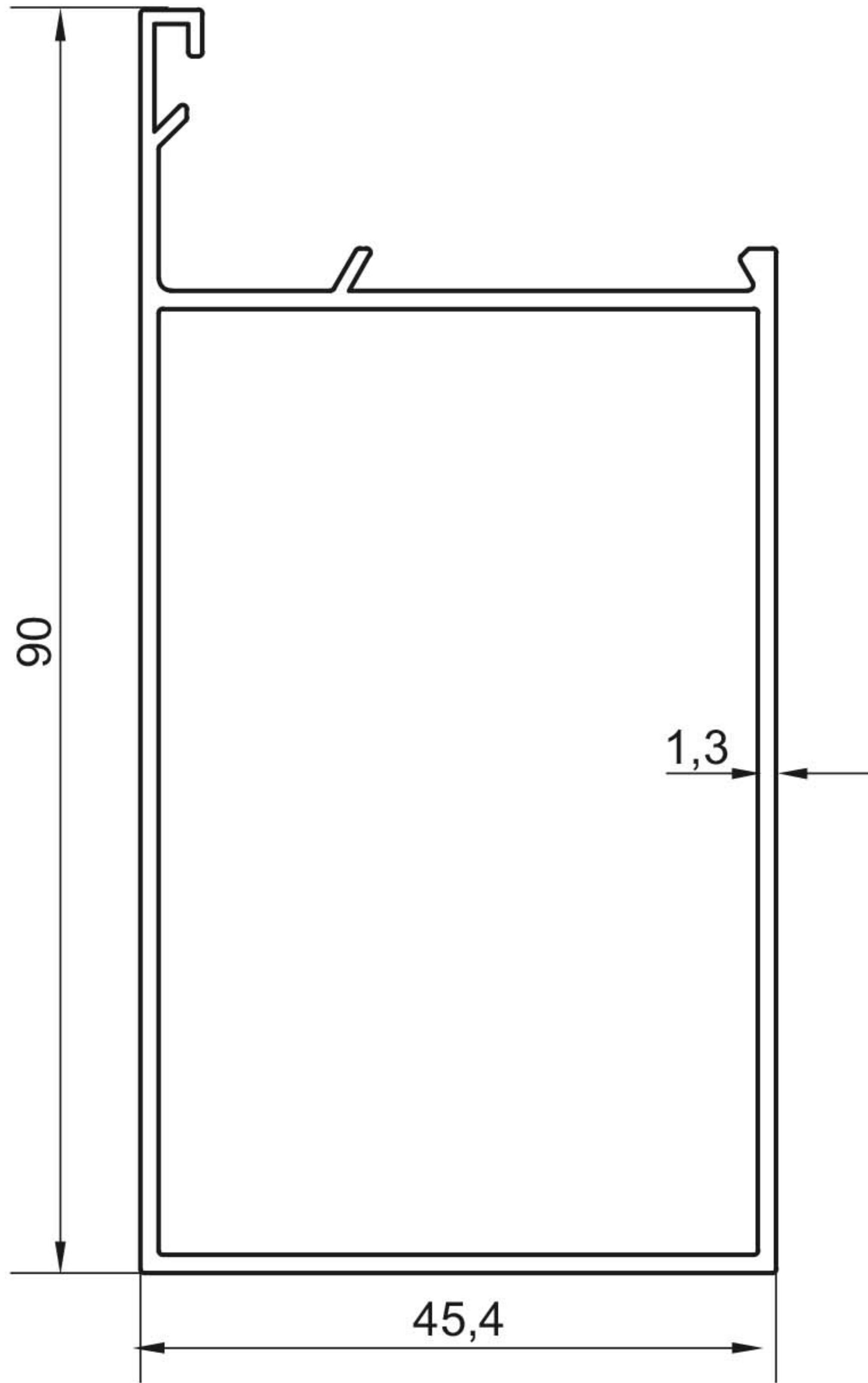
K-2055 908 gr/m
